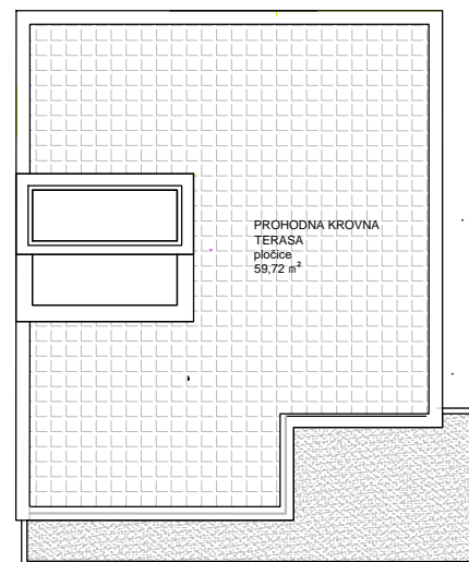
TLOCRT KROVA
