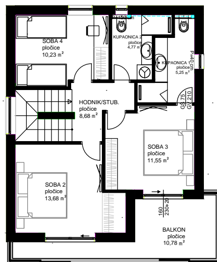
TLOCRT 1. KATA
